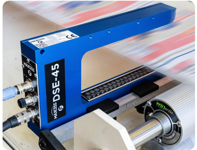
DSE-45 Ultraschallsensor
